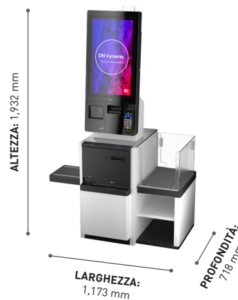
eXpress Max su Cash Rack Altezza: 1,932 mm Larghezza: 1,173 mm Profondità: 718 mm
