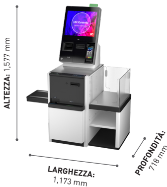
eXpress su Cash Rack Altezza: 1,577 mm Larghezza: 1,173 mm Profondità: 718 mm
